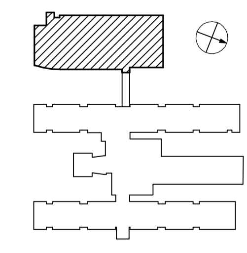
FRAGMENT RZUTU PRZYZIEMIA - APTEKA SZPITALNA TECHNOLOGIA MEDYCZNA SKALA 1:50 Nr rys. 1T
